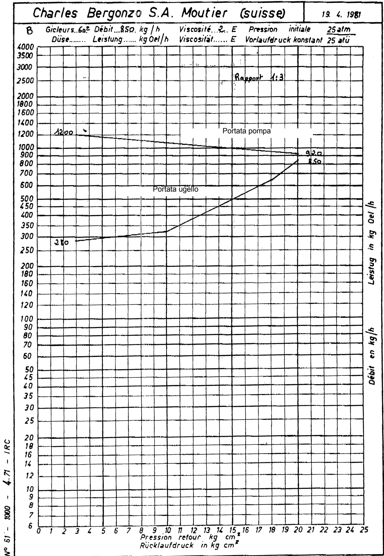
Fig. 16 - Ugello Bergonzo B- Esempio con ugello da 850 kg/h
