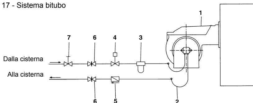
Fig. 17 - Sistema bitubo
