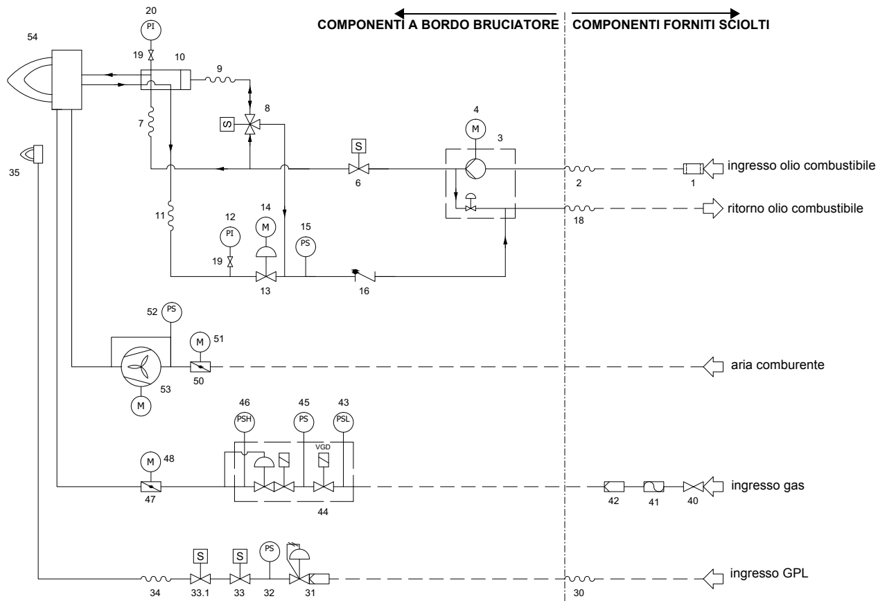
Fig. 4 - 3I2MG-19 v0 Schema idraulico - ugello tipo M3
