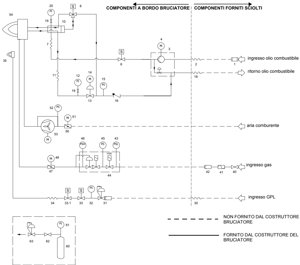
Fig. 5 - 3I2MG-20 v0 Schema idraulico - ugello tipo G, KV
