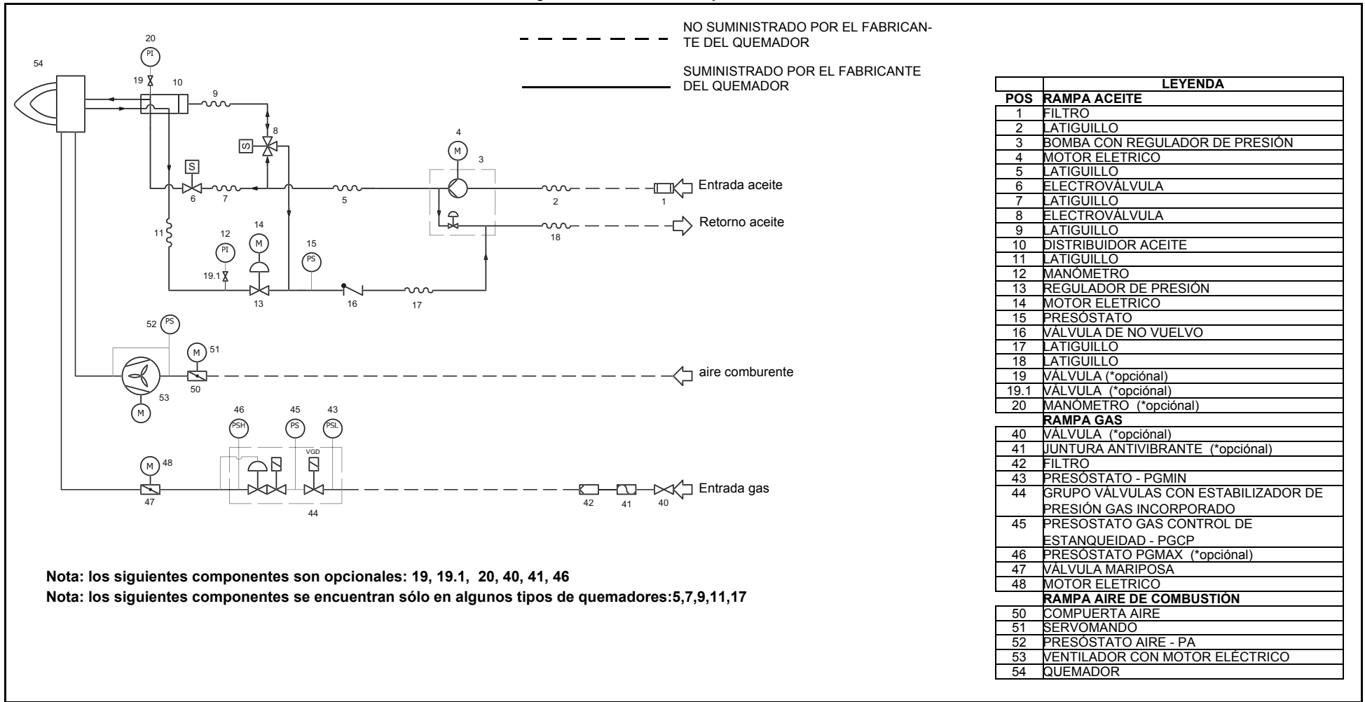
Fig. 2 - 3I2MG-23 v0 Esquema hidráulico
