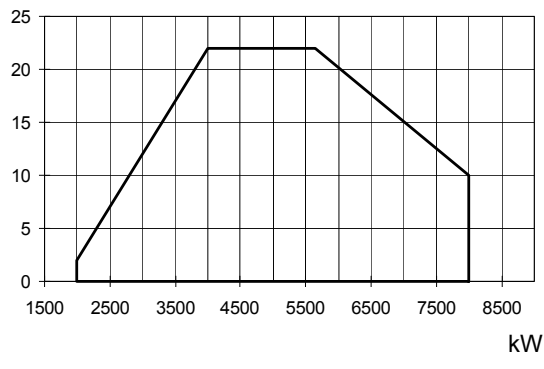
HR525A DN65-80-100
