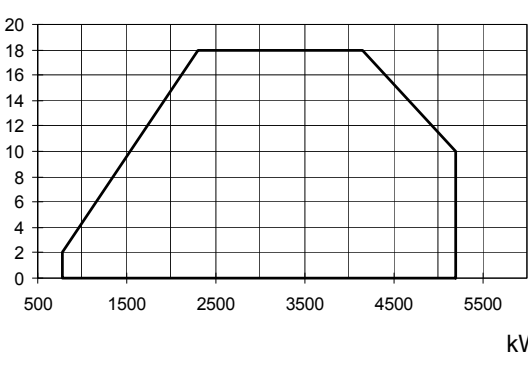
HR525A Rp2
