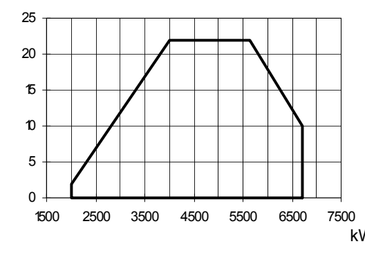
HR525A Rp2
