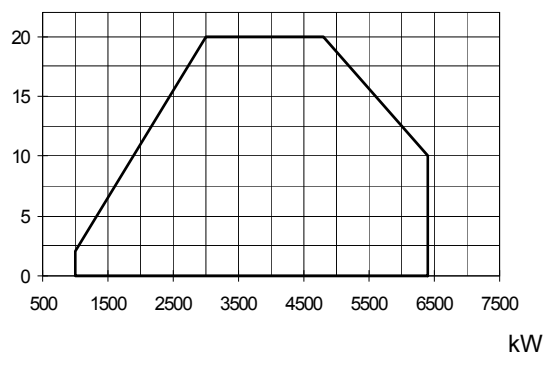
HR525A DN65-80-100
