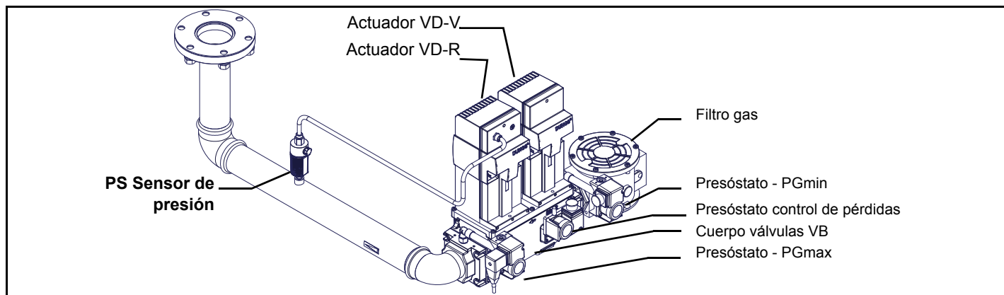
Fig. 15 Ejemplo de rampa gas MBE
