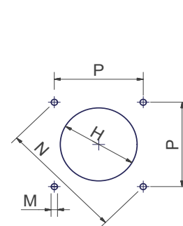
Plantilla de perforación recomendada y brida del quemador
