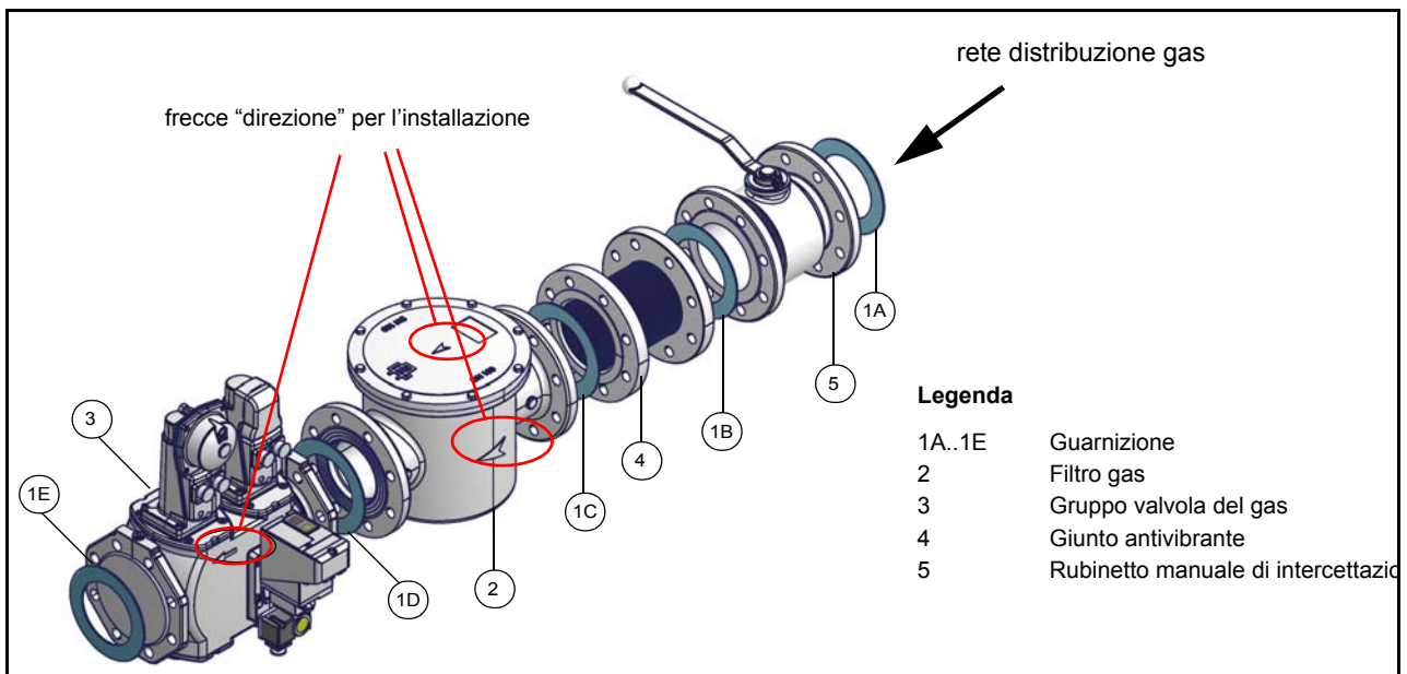
Fig. 6 - Esempio di rampa gas
