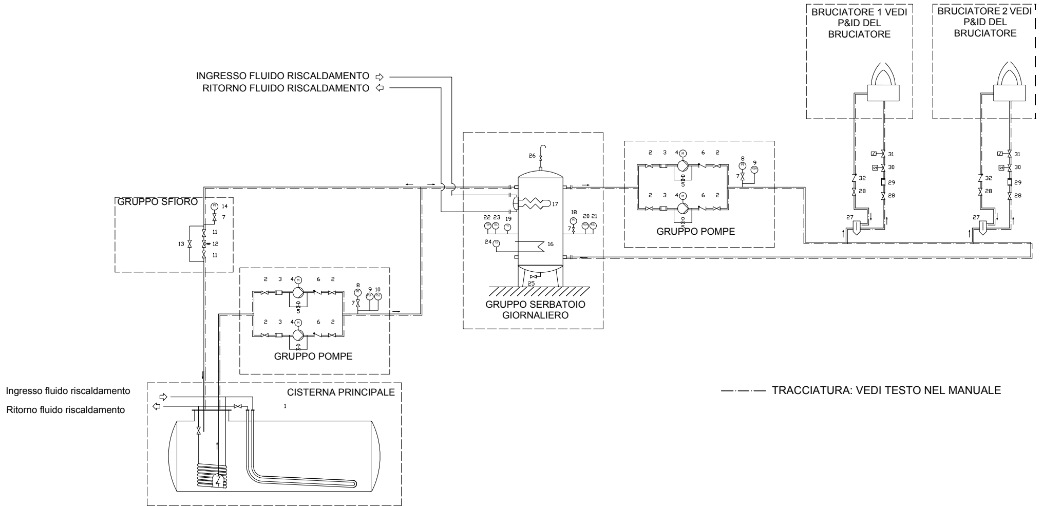
Fig. 13 3ID00014 v2 Schema idraulico - Configurazione per due o più bruciatori
